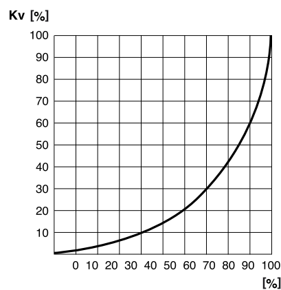
Kv vs. ángulo de apertura en % (agua, 20 °C)
