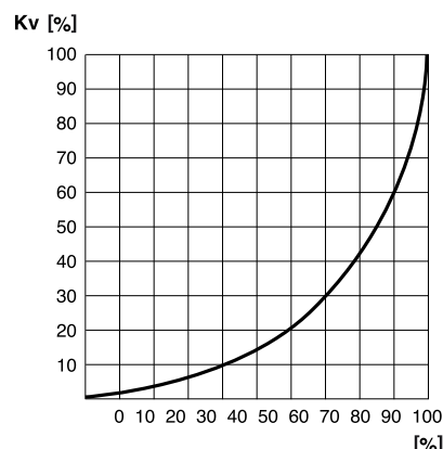
Kv vs. ángulo de apertura en % (agua, 20 °C)
