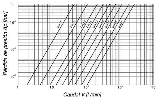
SV 95 : Caudal / Pérdida de presión
